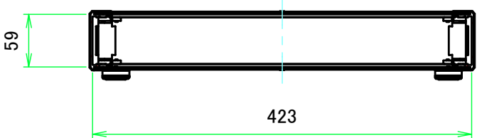
B-B ( 1:6 )
