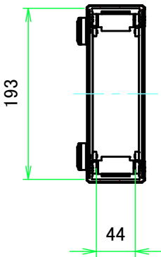
A-A ( 1:6 )
